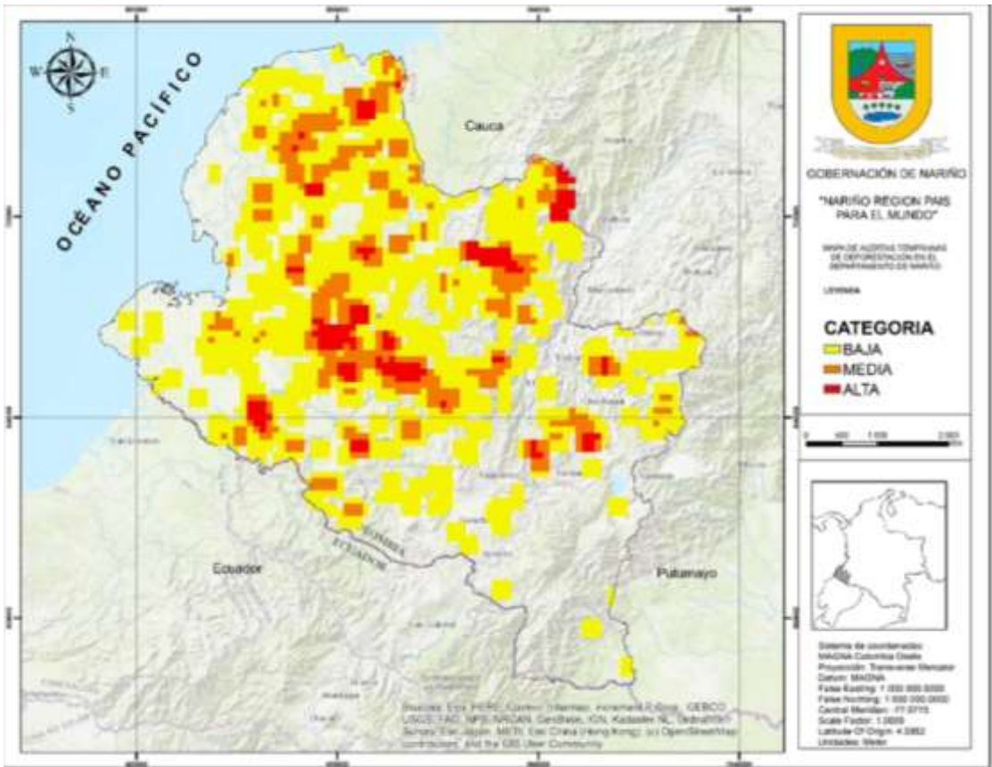
Mapa 32 Alertas tempranas a la deforestación en Nariño
