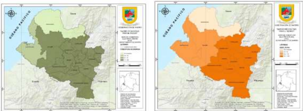
Mapa 17 Cobertura de energía en cabeceras y zonas rurales de Nariño
