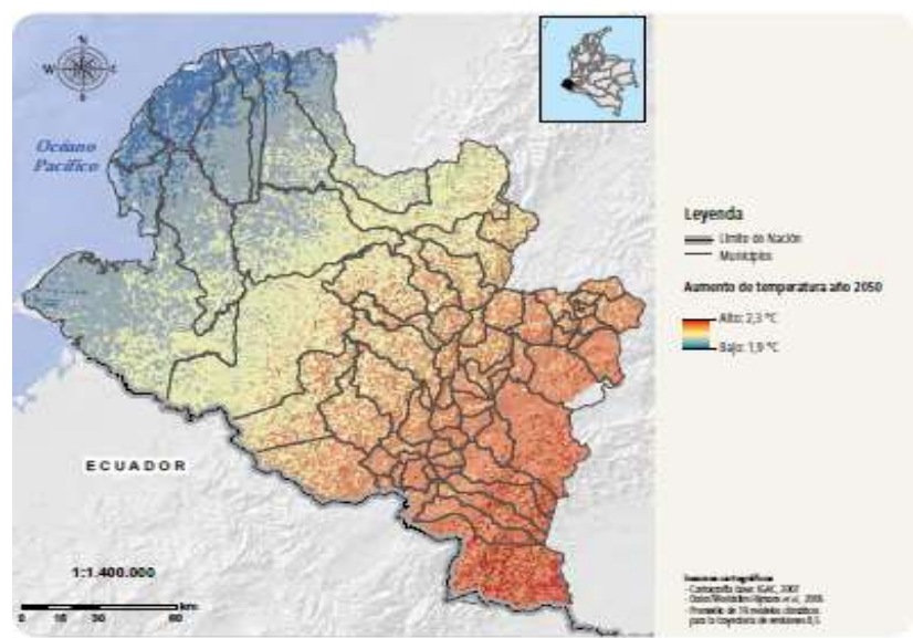
Mapa 33 Cambios esperados en la temperatura de Nariño a 2050
