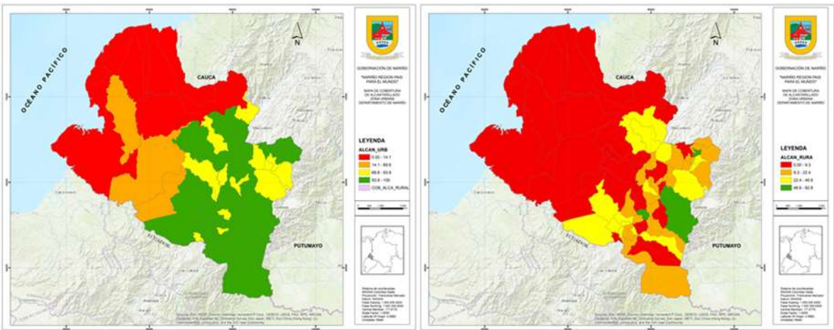
Mapa 14 Cobertura de alcantarillado urbana y rural en Nariño
