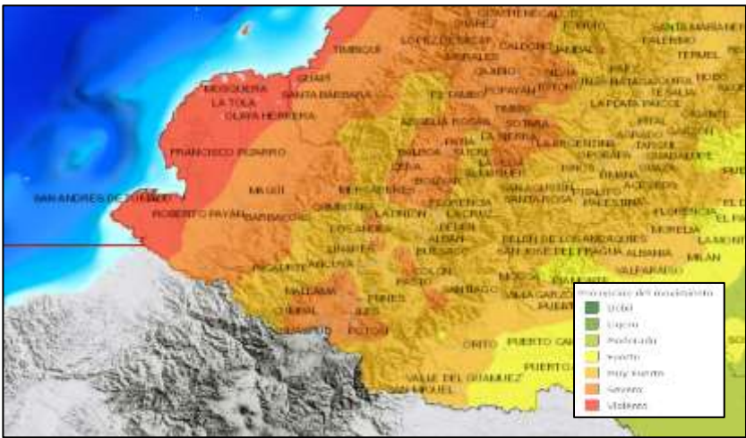
Mapa 42 Intensidad Sísmica del Departamento de Nariño
