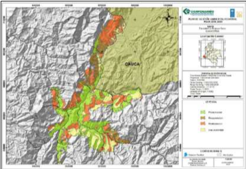
Mapa 46 Zonificación del Ecosistema Seco del Valle del Patía
